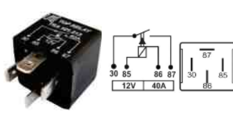
RELE AUX 12V 4T 4A INVERTIDO S/SUPOORTE TRA101213
