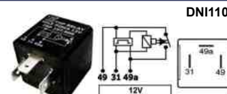
RELE SETA UNIVERSAL 3T BAIXO TRP107000
