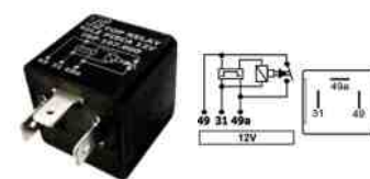
RELE SETA UNIVERSAL 3T BAIXO TRP107000
