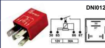
RELE MINI AUX 12V 4T 30A TRA300125
