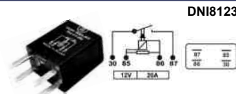
RELE MINI AUX 12V 4T 20A AGULHA TRA811204
